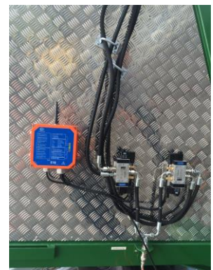
Fernbedienung & Bedienelemente
